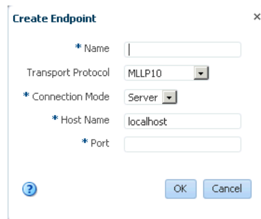
Figure 4-3 Specifying Endpoint Parameters
