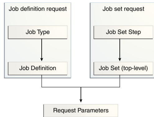
Figure 9-1 Parameter Precedence
