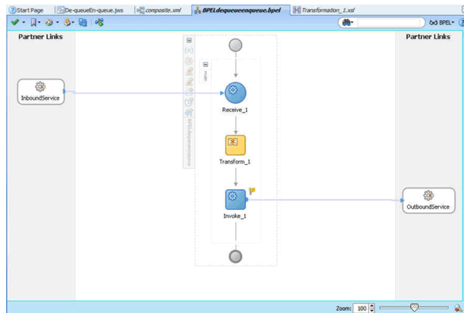
Figure 10-58 The BPELdequeueenqueue.bpel Page
