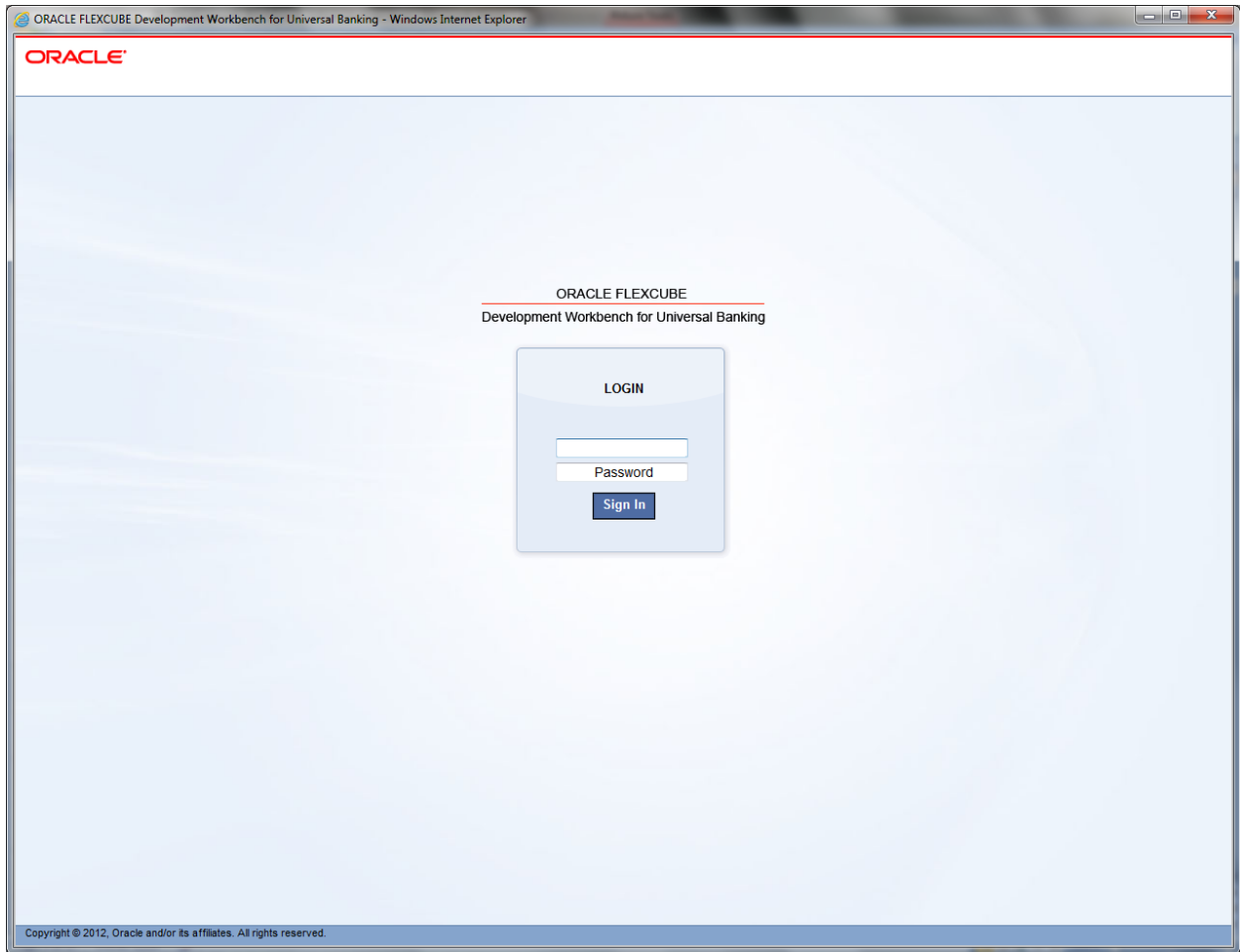
Fig 4.1 Login Page
